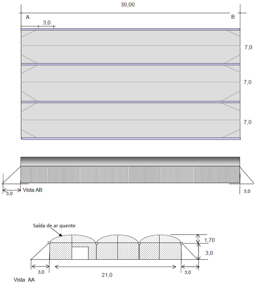
Figura1: Layout sem escala da estufa.
